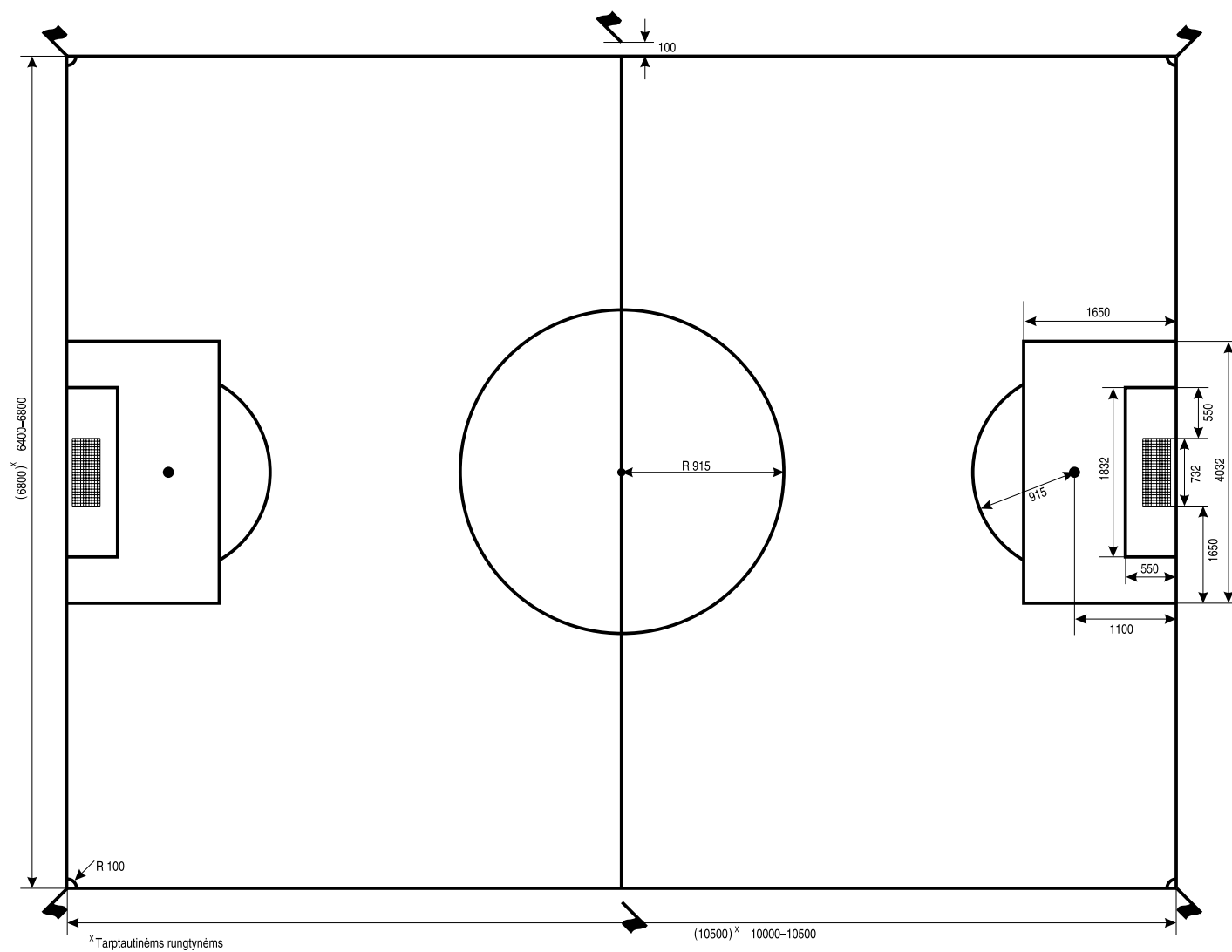
1 pav. Futbolo aikštē
