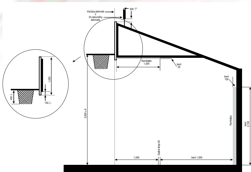
5 pav. Krepšio stovo matmenys
