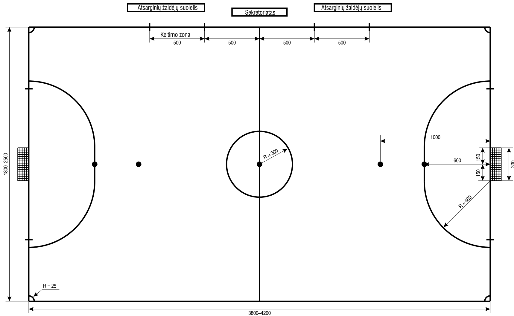
1 pav. Salės futbolo aikštė
