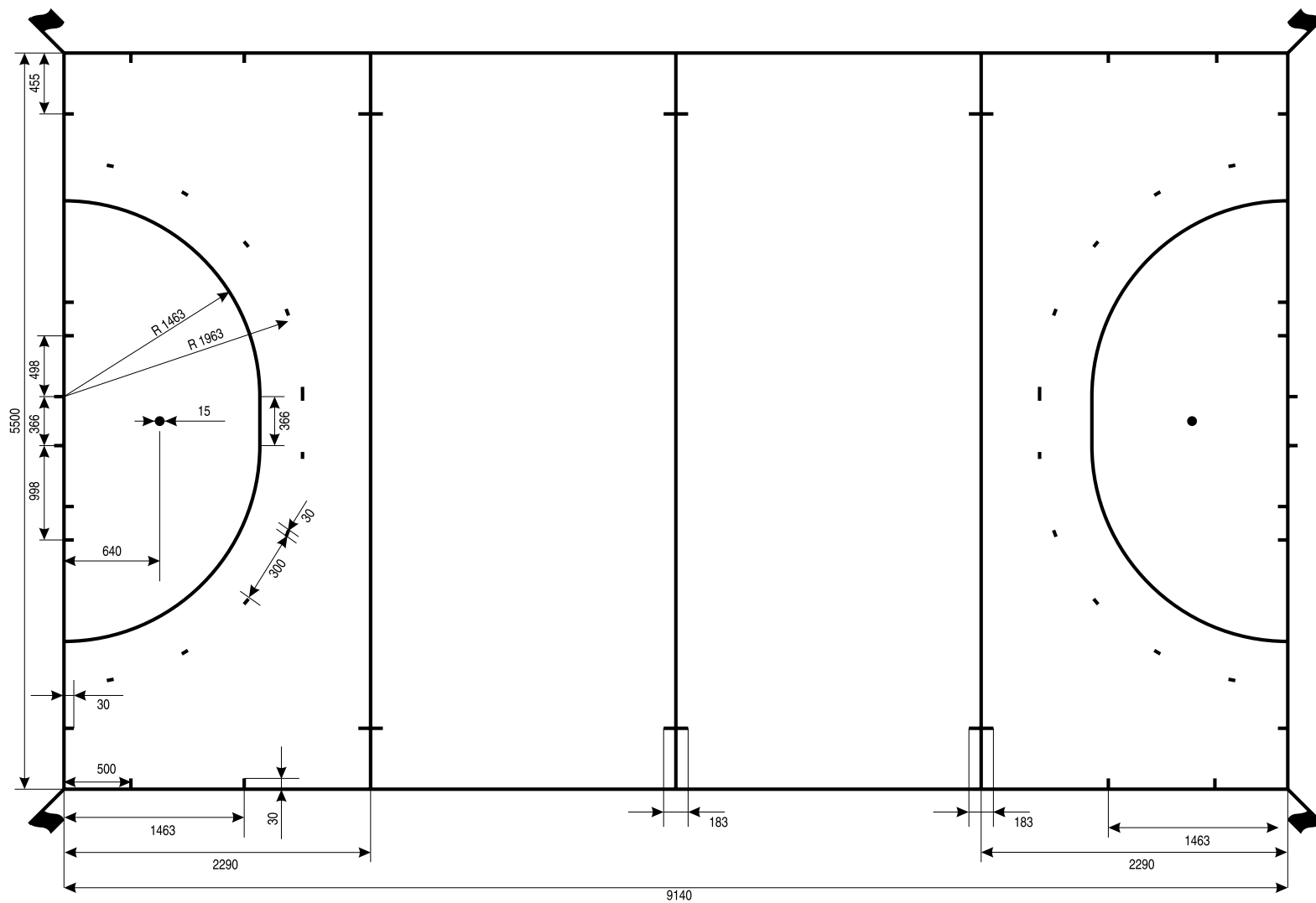
2 pav. Žolės riedulio aikštė
