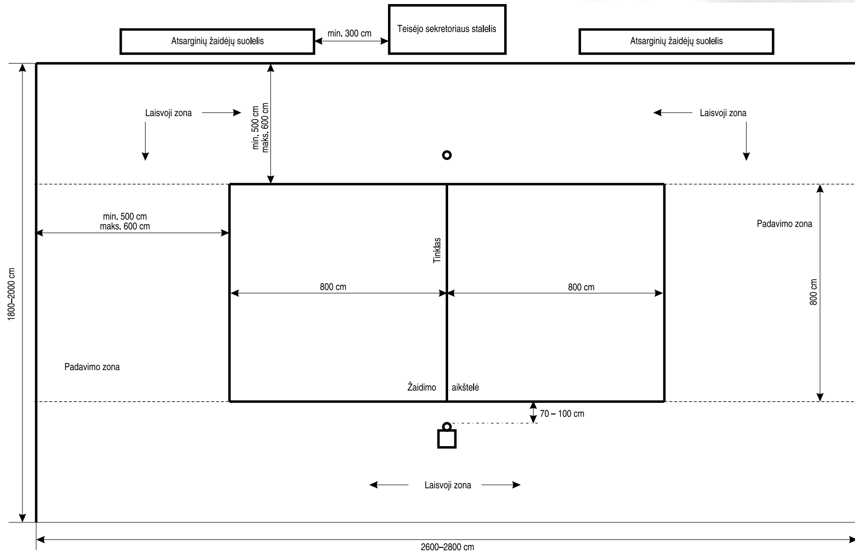
1 pav. Paplūdimio tinklinio aikštelė
