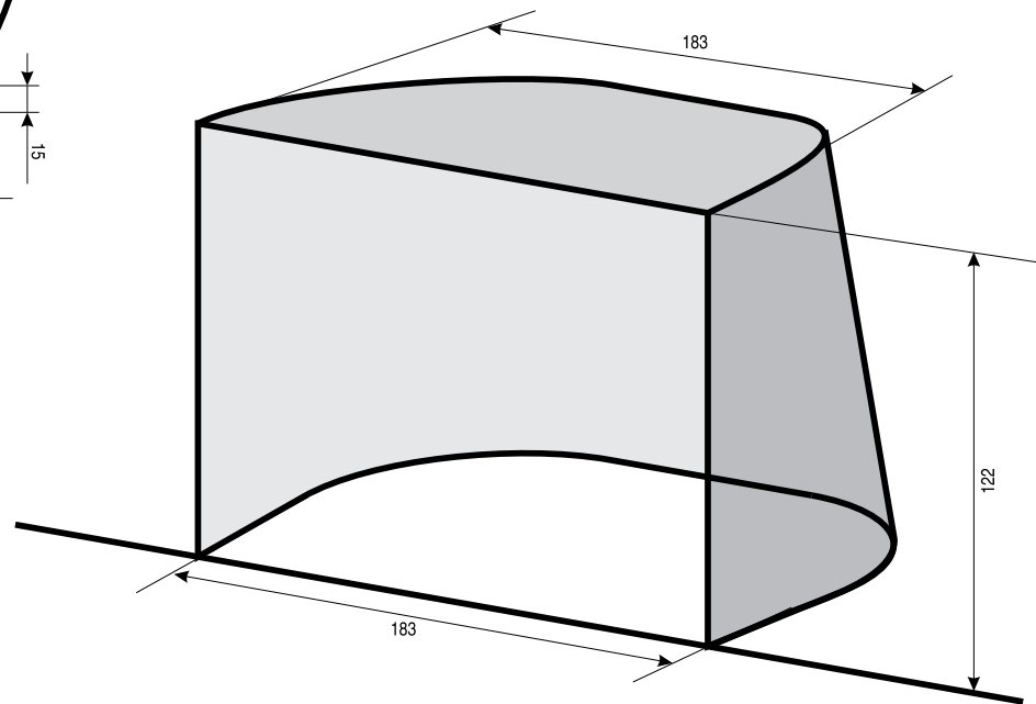
2 pav. Ledo ritulio vartai
