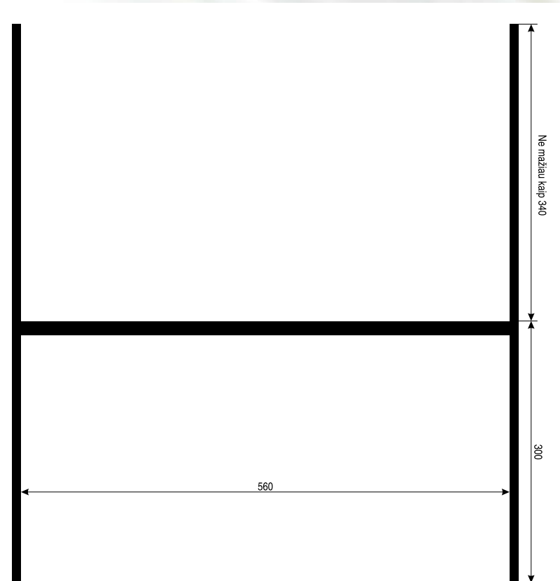
1 pav. Regbio vartai
