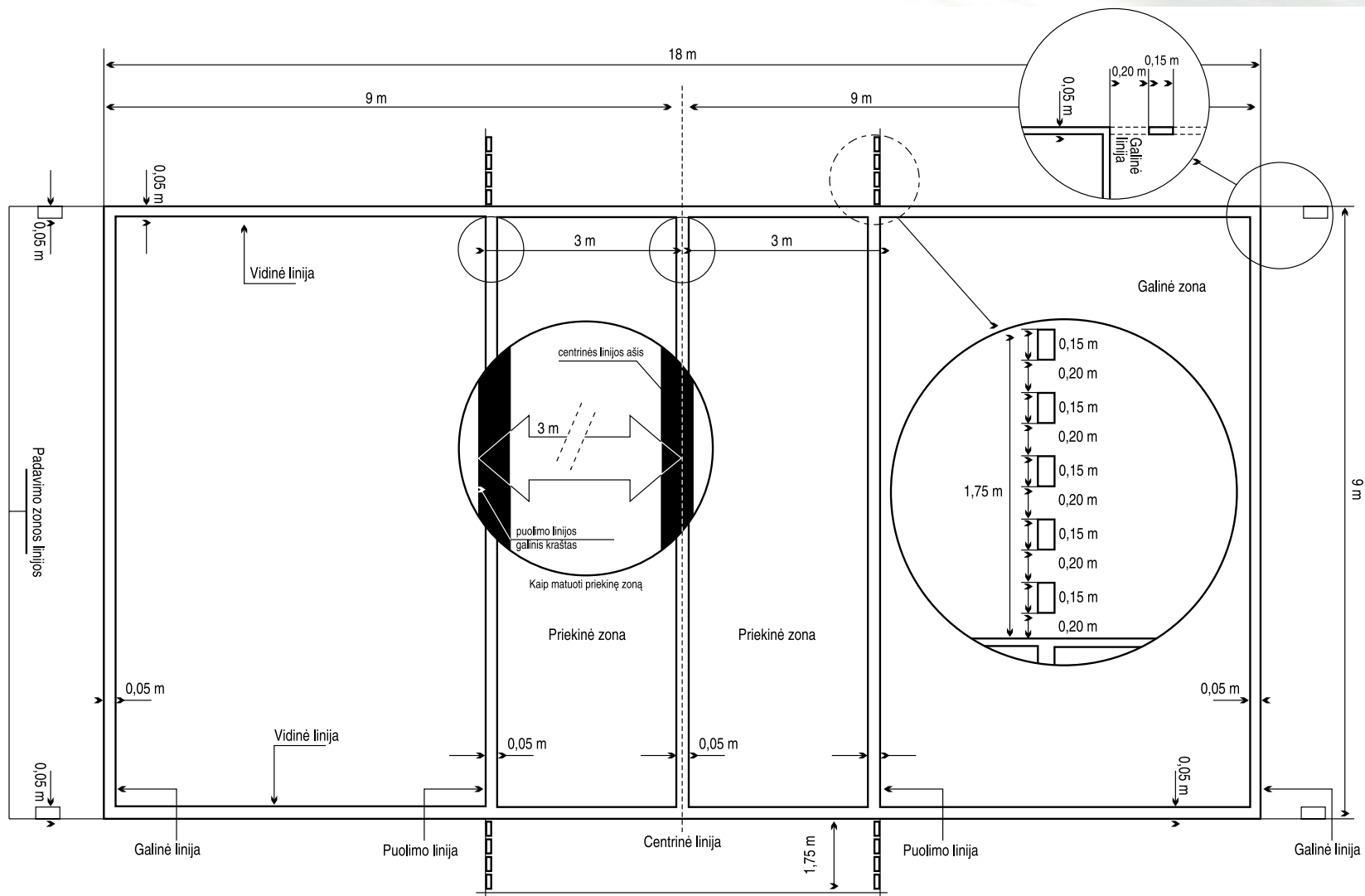
1 pav. Tinklinio aikštelė
