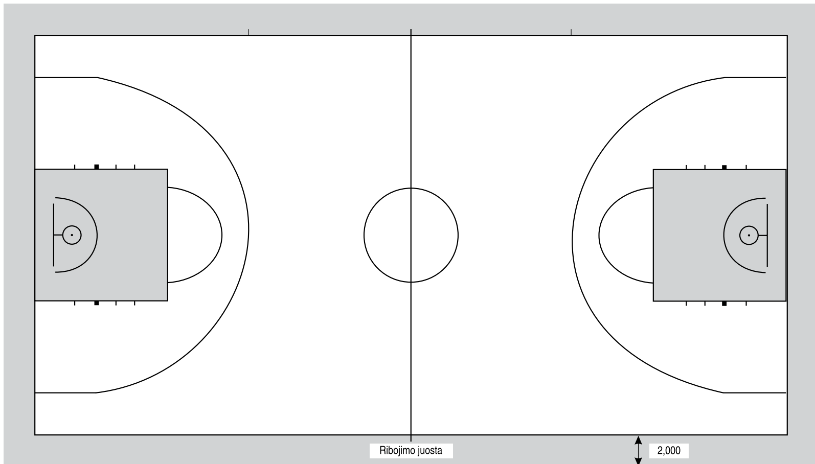
8 pav. Krepšinio rungtynių aikštė
