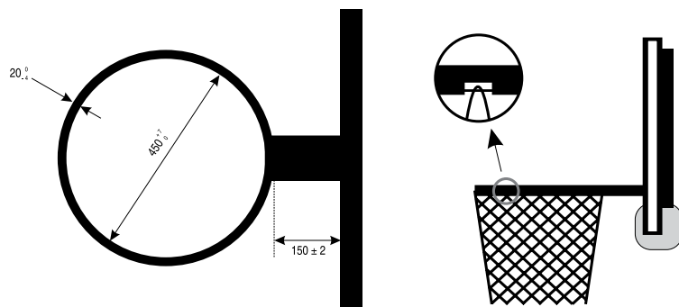
7 pav. Lanko įrenginio matmenys
