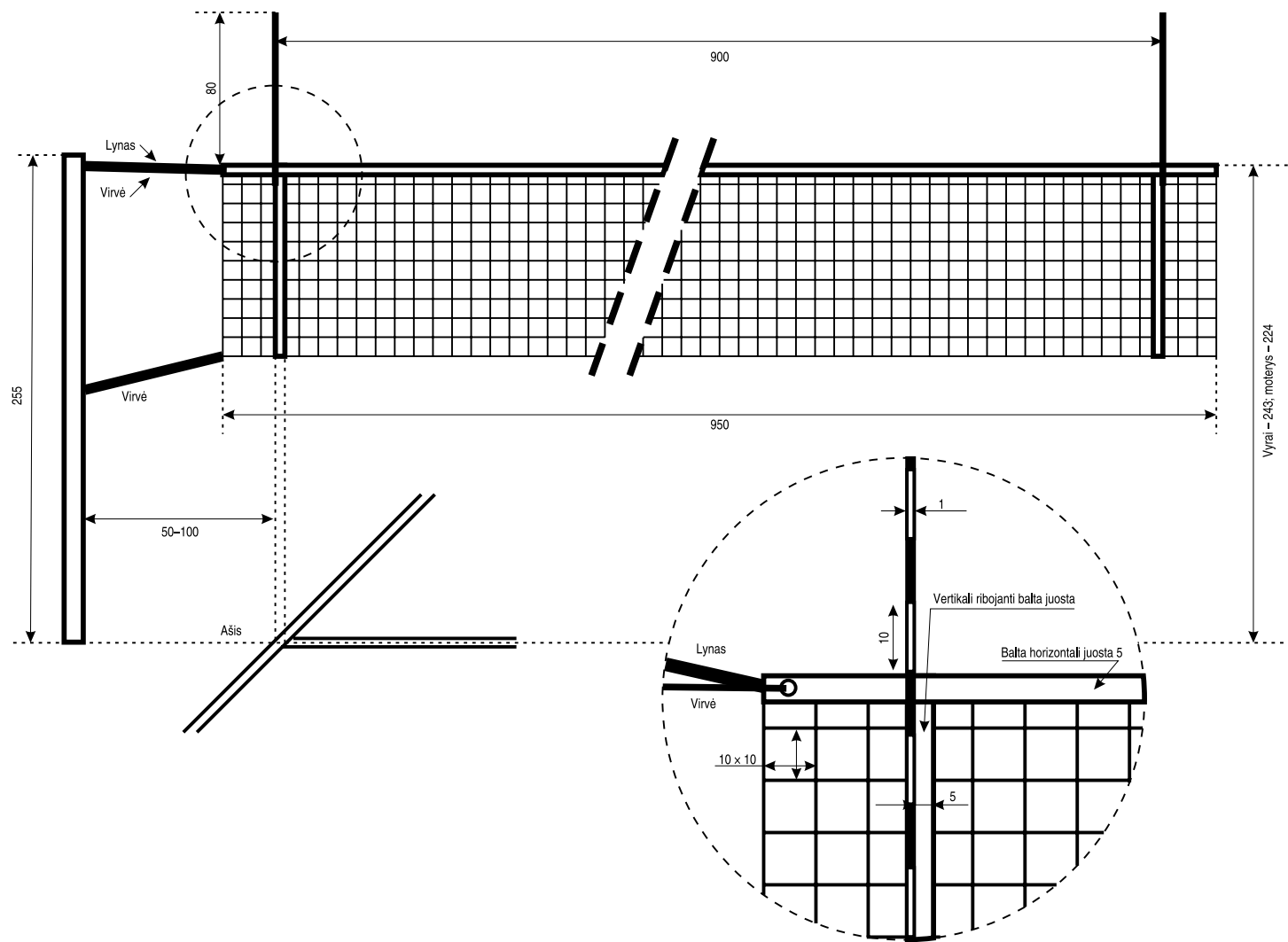
2 pav. Tinklinio tinklas
