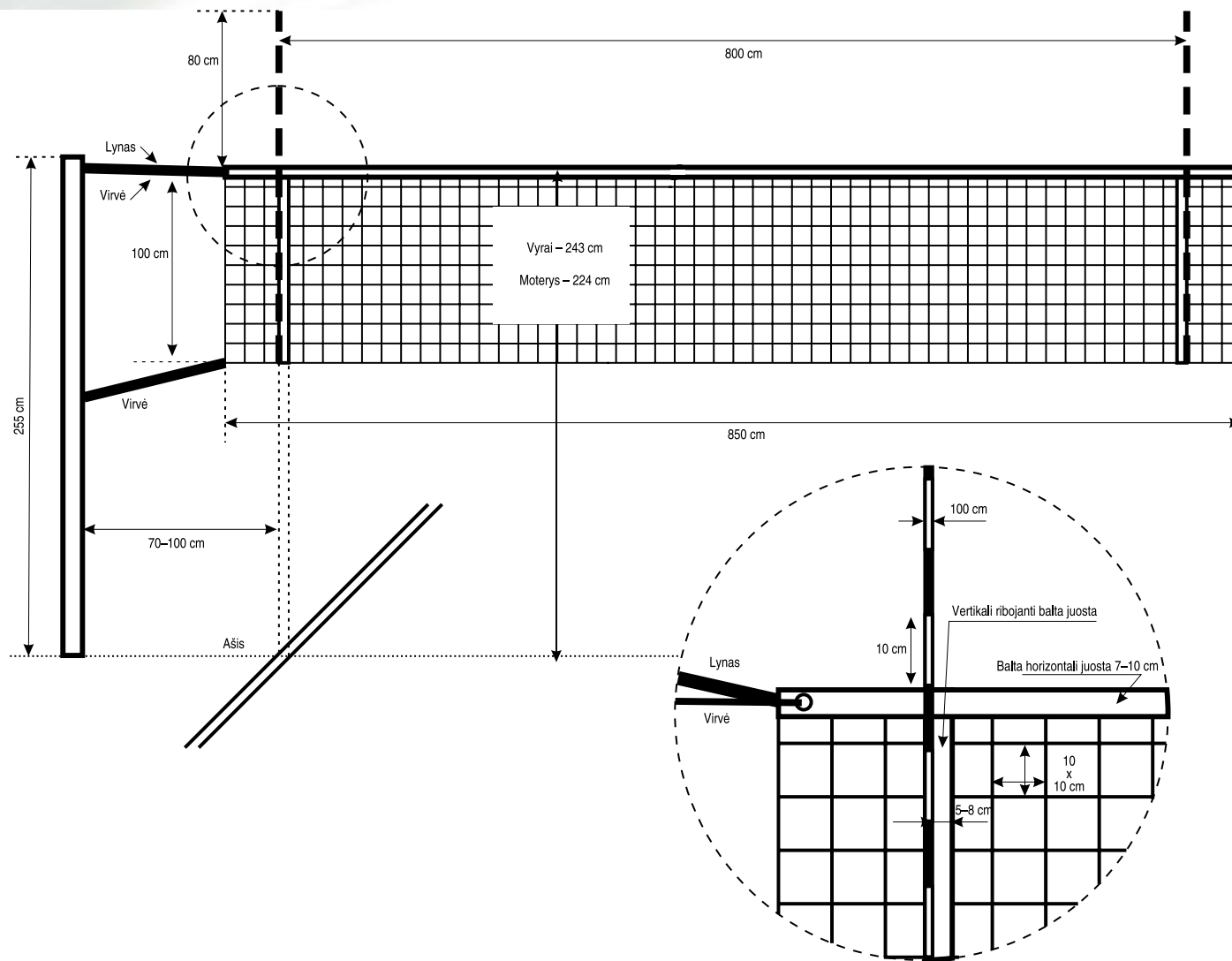
2 pav. Paplūdimio tinklinio tinklas
