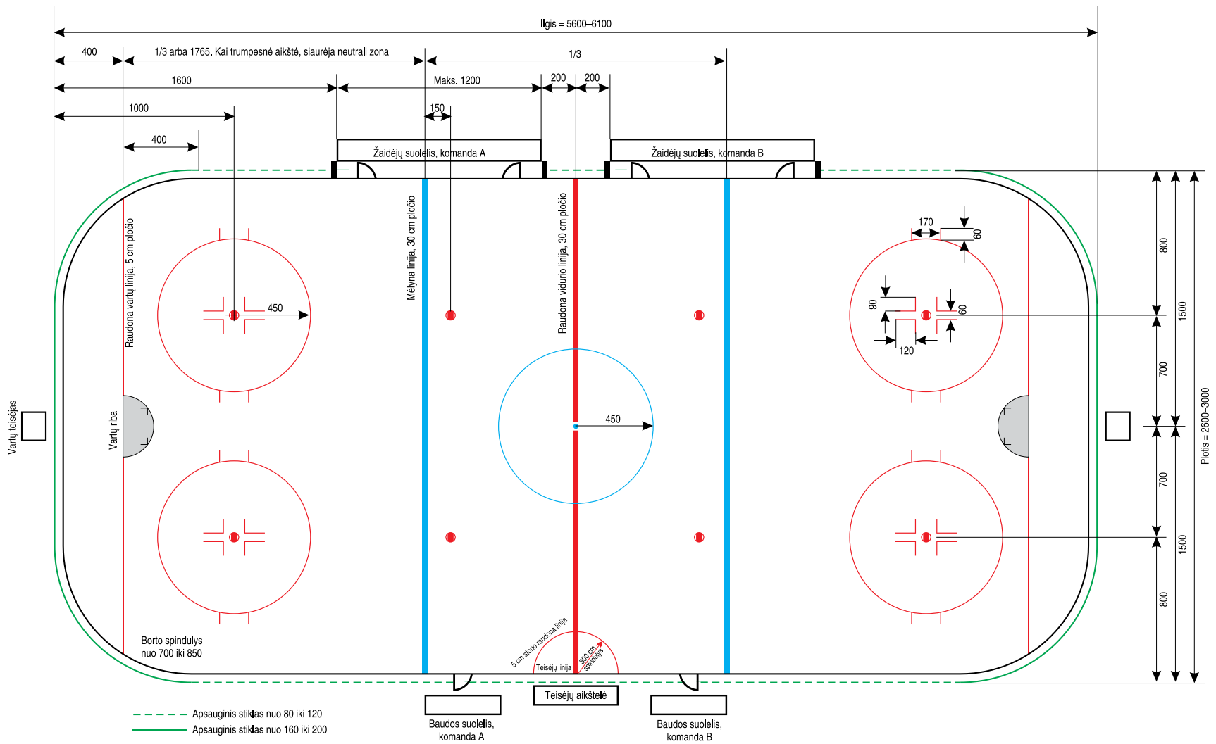
1 pav. Ledo ritulio aikštė
