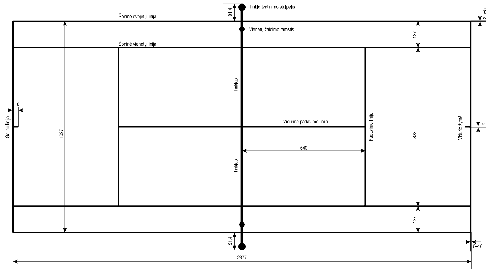
1 pav. Teniso aikštė
