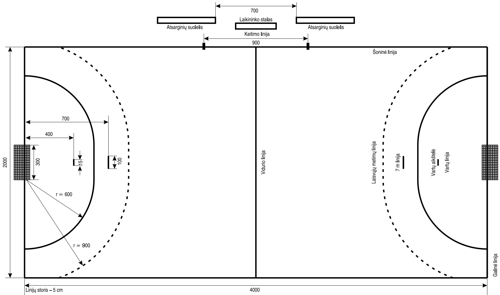
2 pav. Rankinio aikštė
