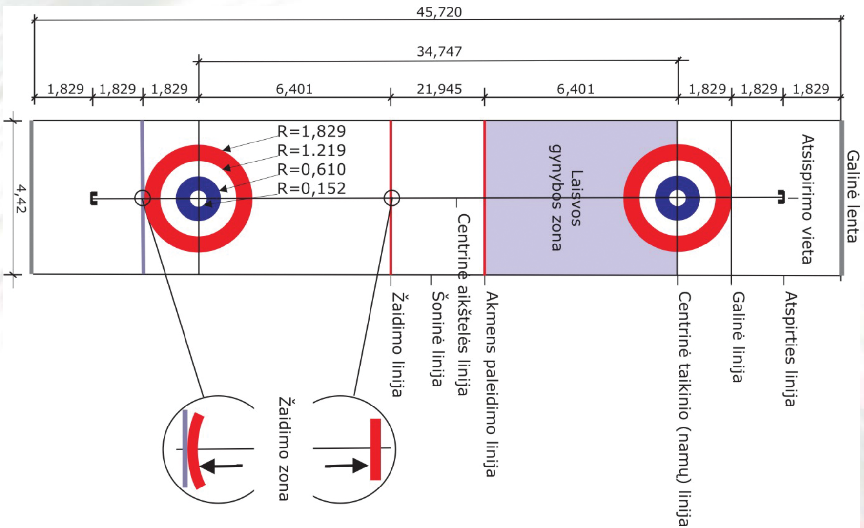
1 pav. Lietuviška kerlingo aikštelė
