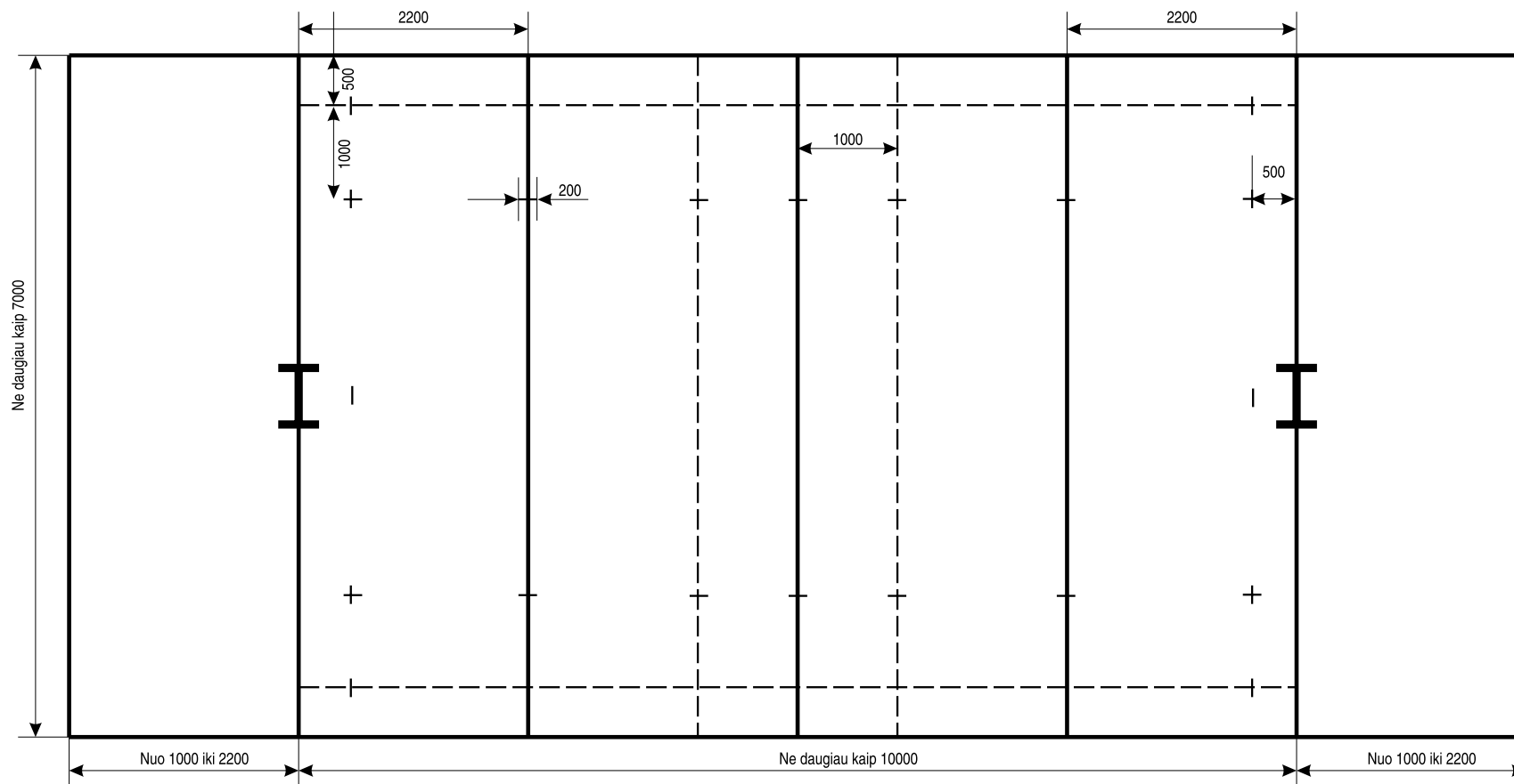
2 pav. Regbio aikštė
