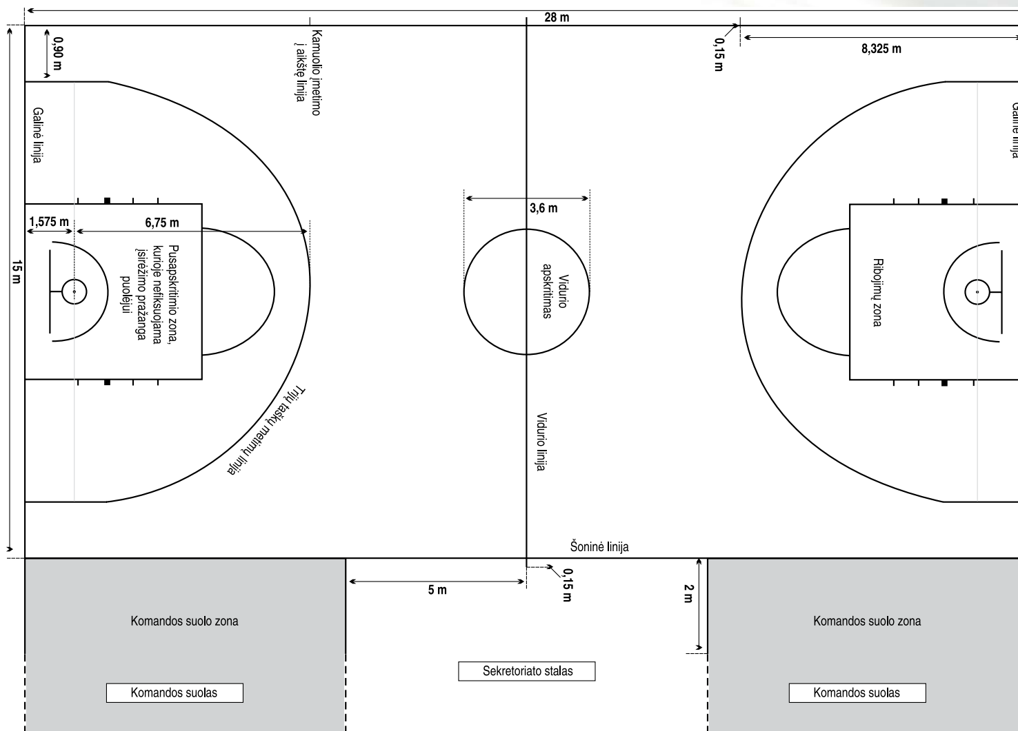
1 pav. Krepšinio aikšlės matmenys
