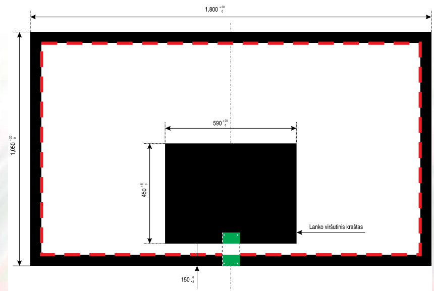
6 pav. Krepšio lentos matmenys
